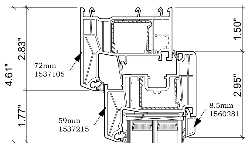
SILL SPACER
