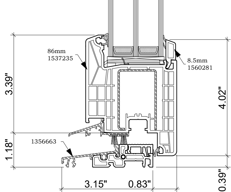
INSWING DOOR
