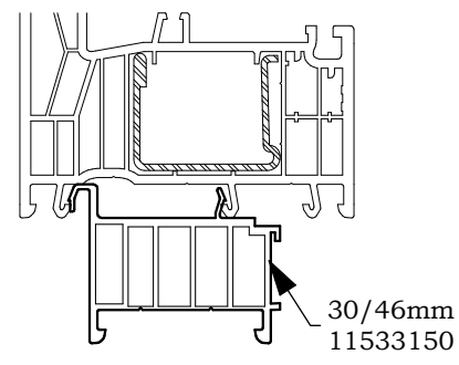
SILL SPACER
