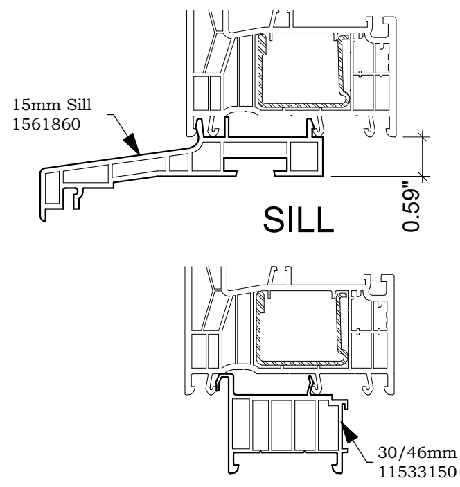
SILL SPACER
