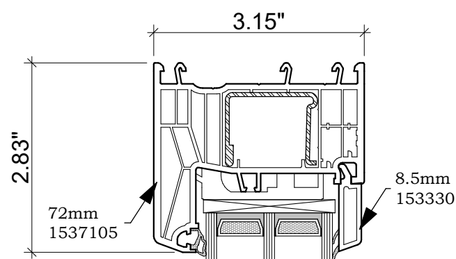
SILL SPACER
